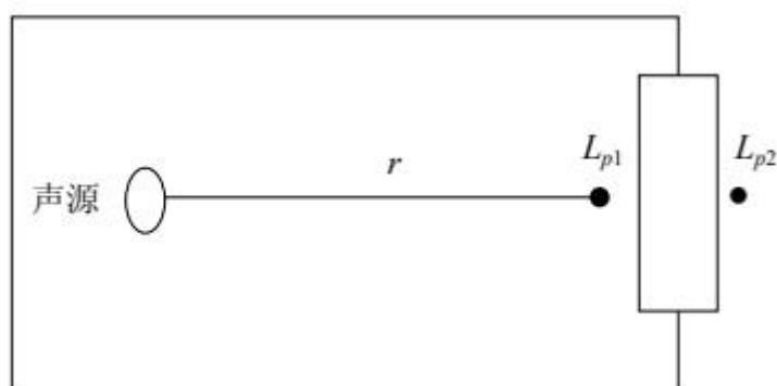
图6-1 室内声源等效为室外声源图例
