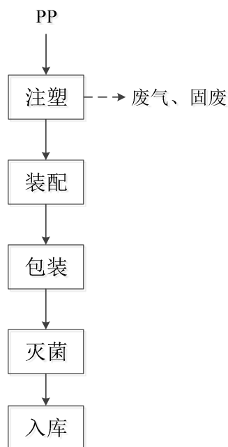
图 1-4 拟建项目 PCR 系列生产工艺流程图（噪声伴随整个工艺流程）
