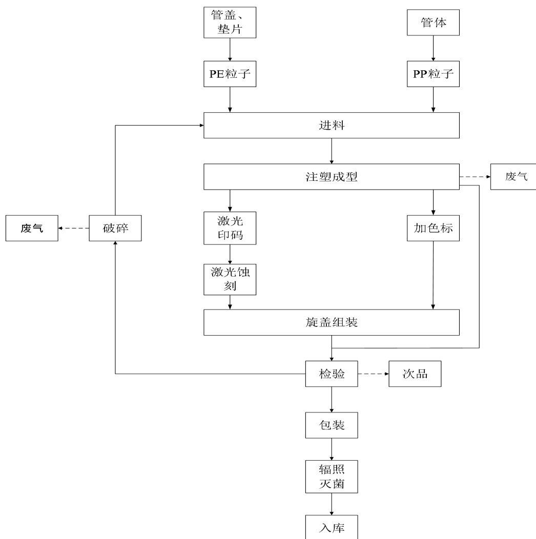
图 1-3 拟建项目冻存管系列生产工艺流程图（噪声伴随整个工艺流程）
