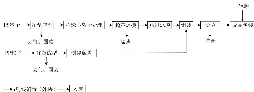
图 1-5 拟建项目细胞培养系列生产工艺流程图（噪声伴随整个工艺流程）
