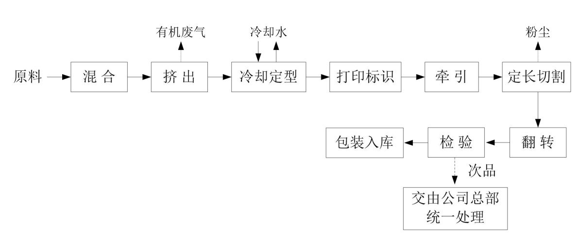
图 1-1 现有项目生产工艺流程及产污环节示意图
