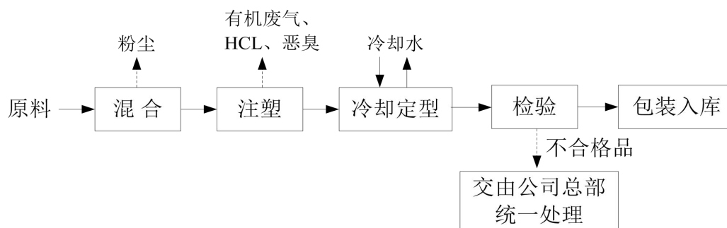
图 4-1 PVC 塑胶管道生产工艺流程及产污环节示意图
