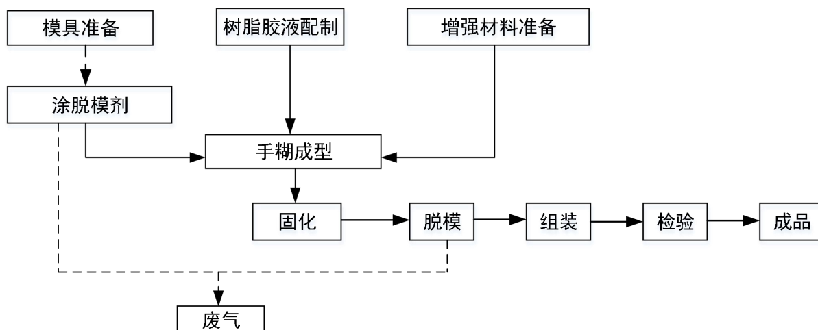
图 4-3 机身生产工艺流程图
