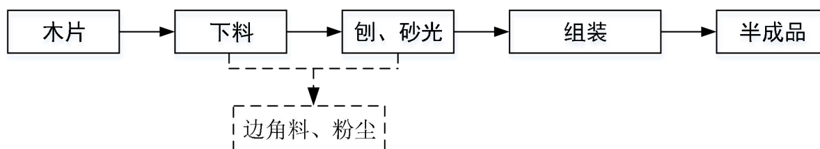
图 4-1 木配件生产工艺流程图
