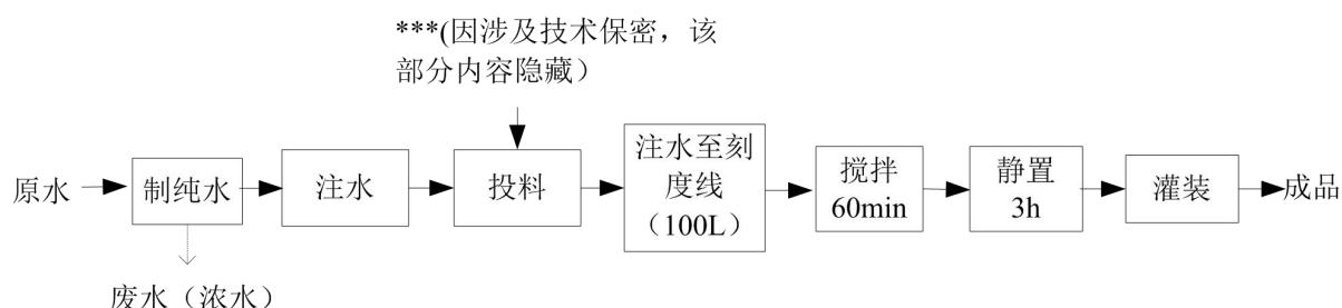
图 4-1 项目产品生产工艺流程及产污环节示意图
