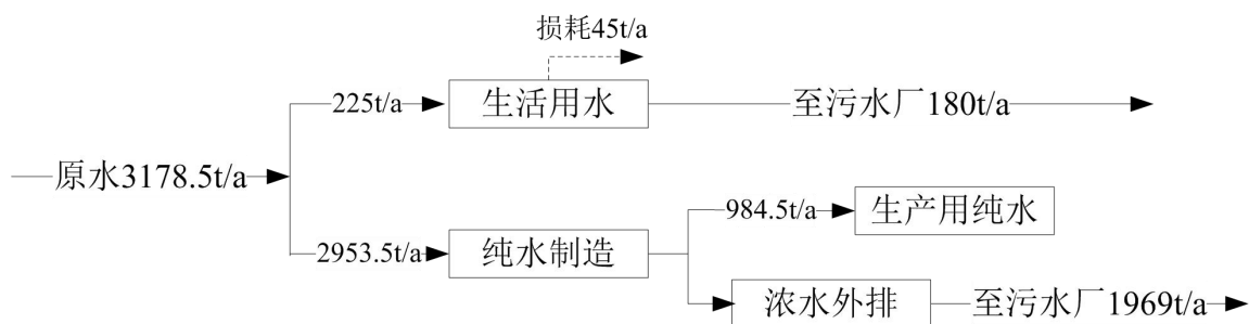
图 4-2 项目水平衡图
