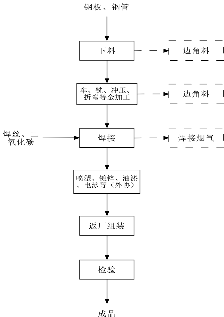
图 4-1 本项目生产工艺情况图（噪声伴随整个生产过程）
